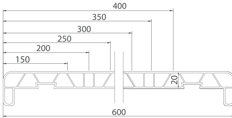
Denizlik PVC Sill
