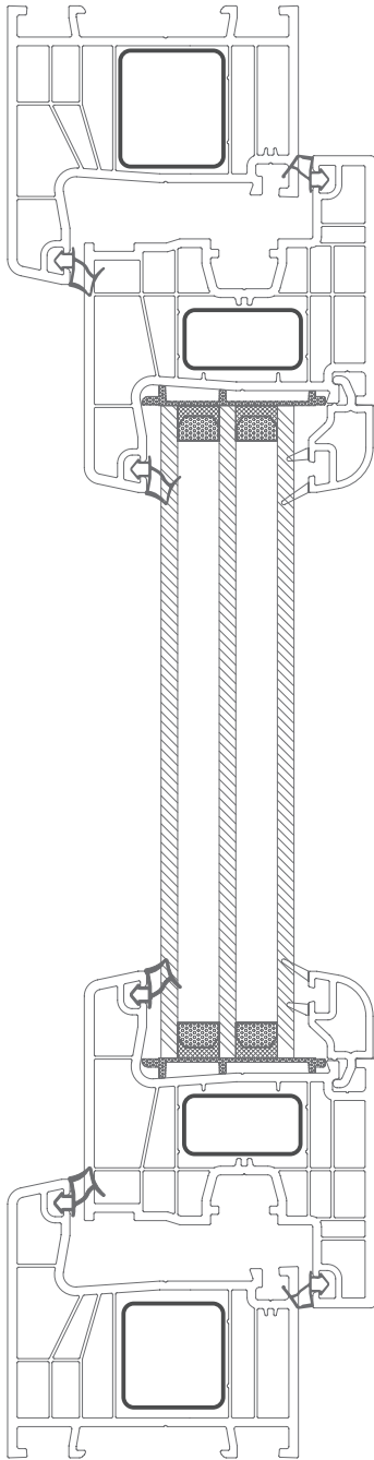
A-A KESİTİ
