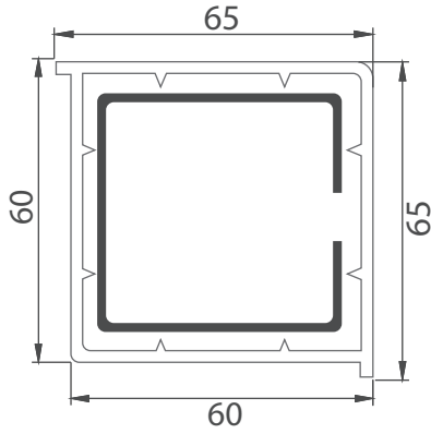
60 mm Köşe 60 mm Corner Box
