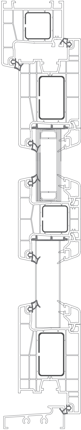
A-A KESİTİ
