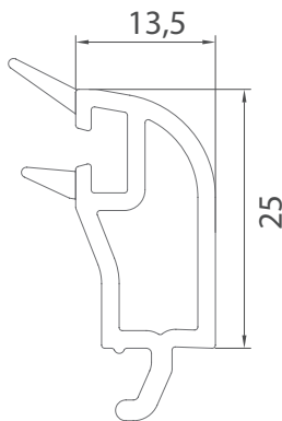
Energy 44 mm Üç Cam Çita Energy Triple Glazing Bead 44 mm
