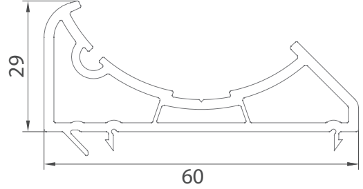
Boru Adaptörü Pipe Adaptor
